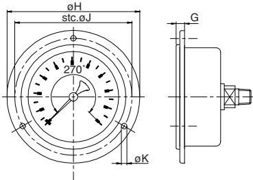
7016 frontflange
