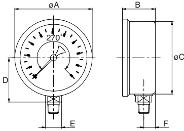
7011 bottom
